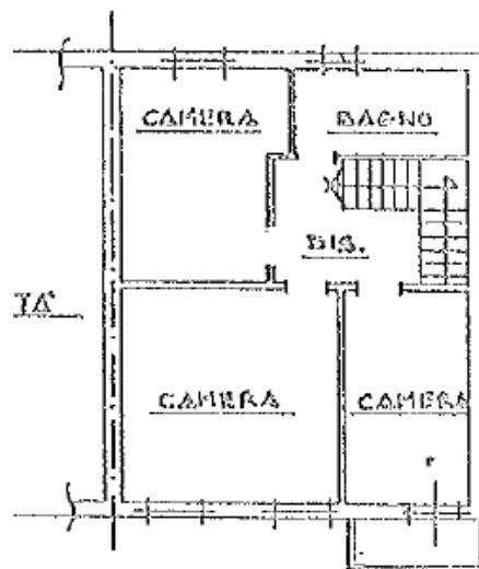
PIANO PRIMO h=2.75 m
