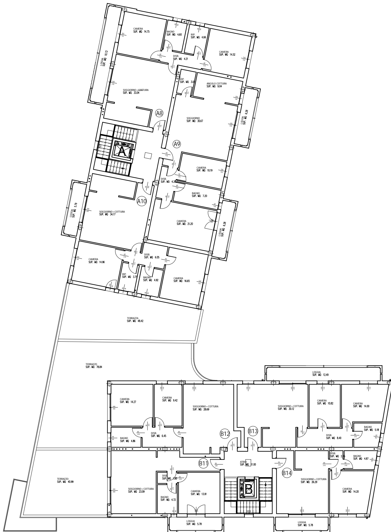
PIANO SECONDO
